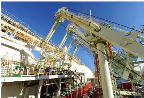
TBG 製 ローディングアーム
